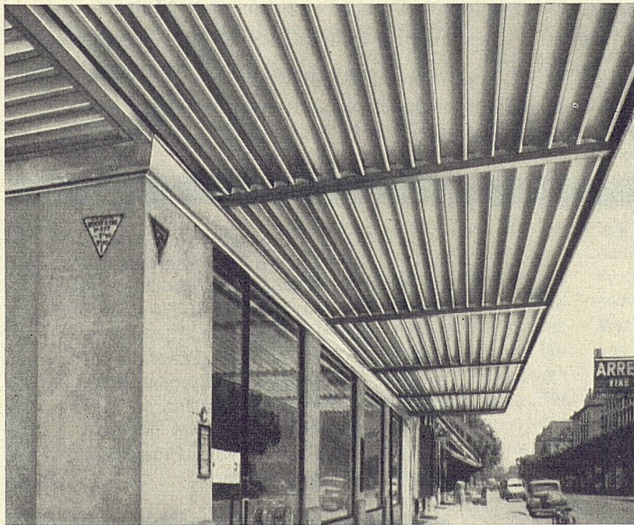
Schaufenstervordach der Pharmacie Bédat, Genf Architekt: Maurice Cailler, Genf
