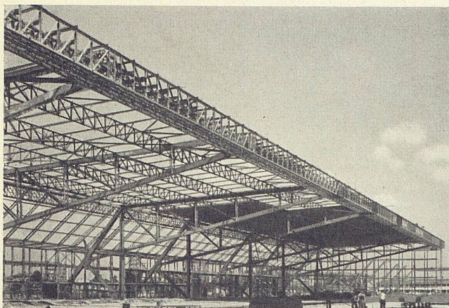
1 Empfangsgebäude Flughafen Orly-Paris
