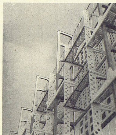
2 Hangar in Stahlkonstruktion, Flughafen Orly-Paris
