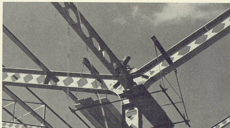
3 Eingangsfront der Messehalle in Lille Konstrukteur: Jean Prouvé
