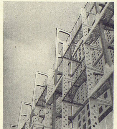
2 Hangar in Stahlkonstruktion, Flughafen Orly-Paris
