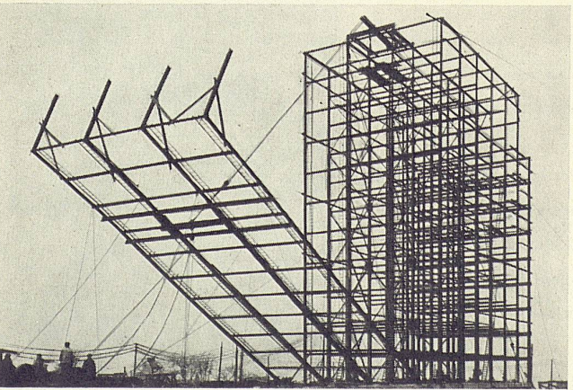
4 Konstruktion einer Kunsteisbahn in Paris
