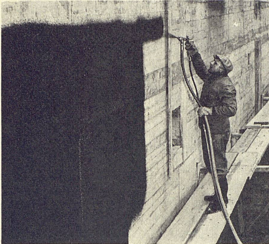
Fundamentabdichtung am neuen Verwaltungsgebäude des Elektrizitätswerkes Winterthur
