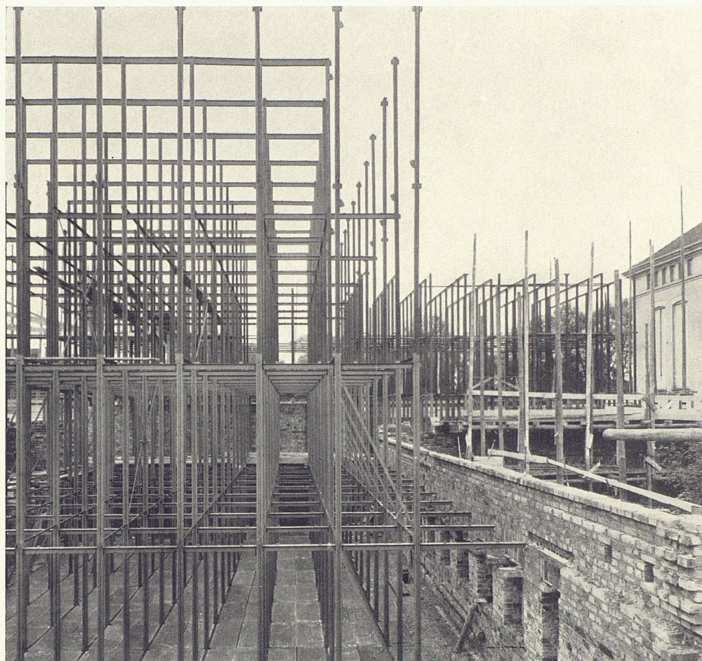
Eine 12-geschossige Bibliotheksanlage für die Universität Gießen ist gegenwärtig im Bau
