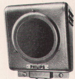
6 W-Schrägstrahler EV 5705 für Sprach- und Musikübertragung
