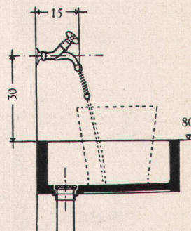
Wandbatterie 1375/150 Neo mit Schlauch 1375/150 S Neo
