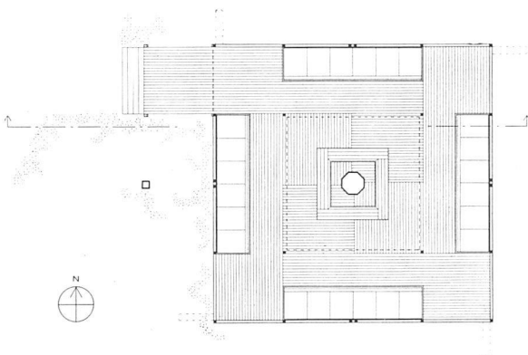
Grundriß: 1:300 | Plan | Lay-out
