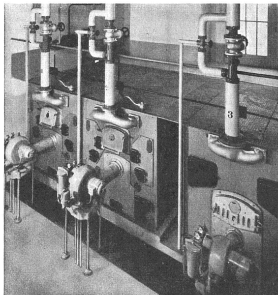
Fern-Heizzentrale mit 3 Großkesseln und Schwerölf Feuerungen
