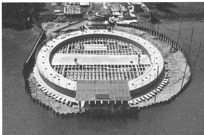
Schwimmendes Nichtschwimmerbecken Ø 27 m in armiertem Beton, während der Bauausführung im Trockendock
