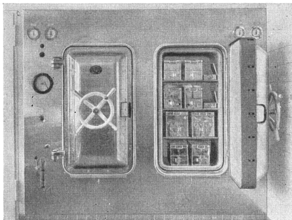
Abbildung: Anlage im Stadthospital Waid, Zürich
