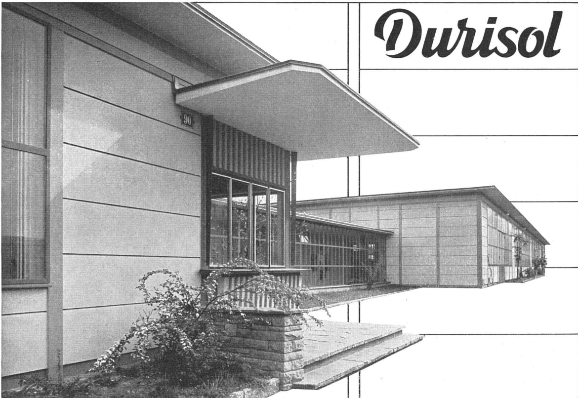
Unterkunftsgebäude und Montagehalle einer Werkzeugmaschinenfabrik in Zürich Durisol-Aussenwandplatten 10 cm stark und Durisol-Dachplatten
