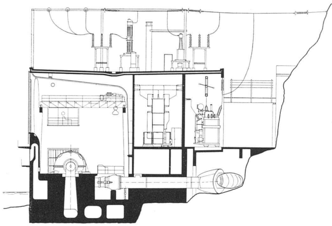
Querschnitt 1:500 | Coupe | Cross-section
