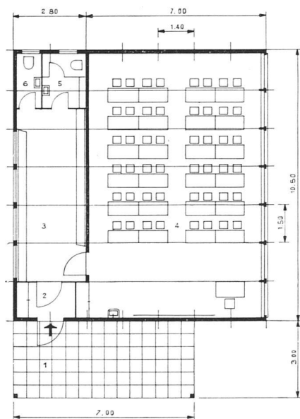
Grundriß 1:200 | Plan
