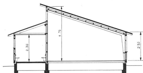
Querschnitt 1:200 | Coupe | Cross-section
