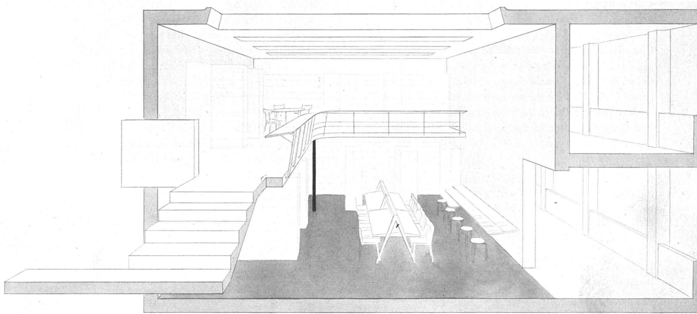
Querschnitt durch Lesesaal mit Galerie / Coupe transversale / Cross section
