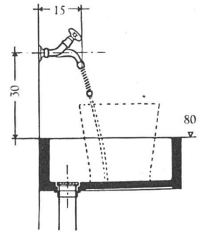
Wandbatterie 4375/150 Neo mit Schlauch 4375/150 S Neo
