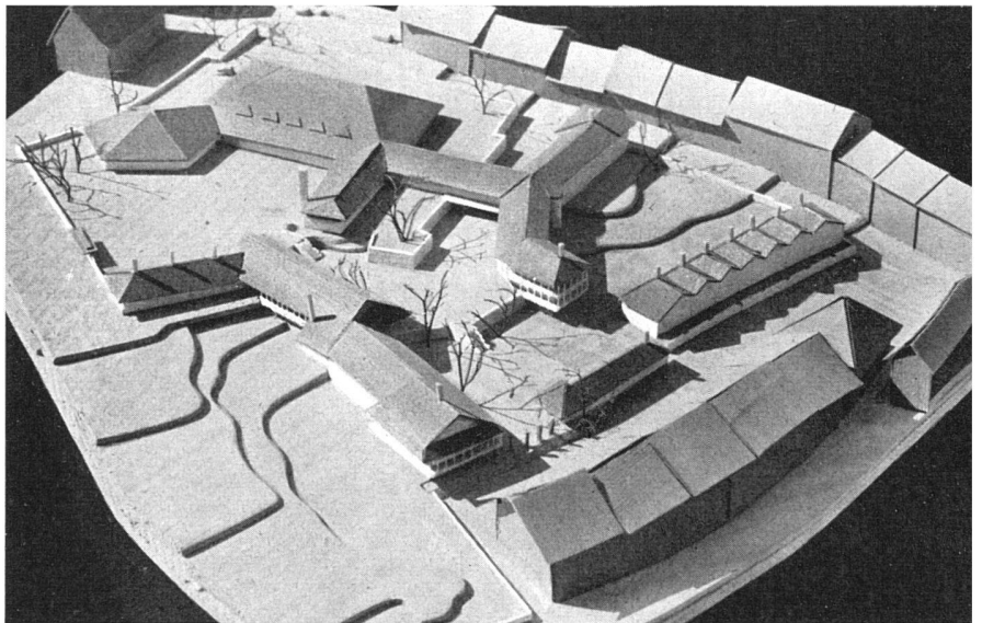
Kunstzentrum mit Saalbau, Klubhäusern, Ateliers. Überbauung des Obmannamt-Areals Zürich in Verbindung mit der Altstadtanierung | Centre d'Art avec salles d'exposition, salles de clubs, ateliers d'artistes | Art Centre, exhibition rooms, club rooms, artist's studios
