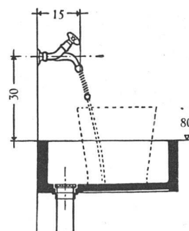
Wandbatterie 4375/150 Neo mit Schlauch 4375/150 S Neo
