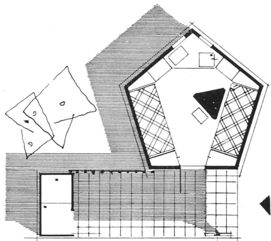
Grundrisse Einzelhaus 1:100 und kombinierte Anlagen 1:200 | Plan | Groundplan detached house and combined lay-outs
