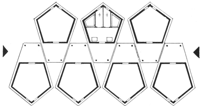
Grundrisse Einzelhaus 1:100 und kombinierte Anlagen 1:200 | Plan | Groundplan detached house and combined lay-outs
