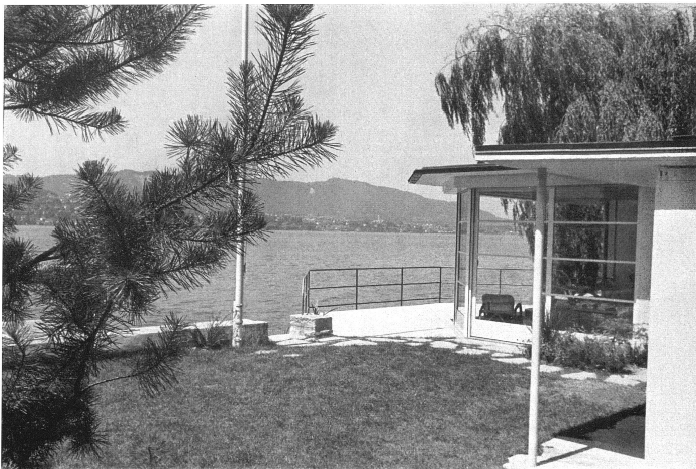
Wochenendhaus in Goldbach, B. & E. Gerwer, Architekten, Zürich | Maison de week-end à Goldbach | Week-end house in Goldbach
