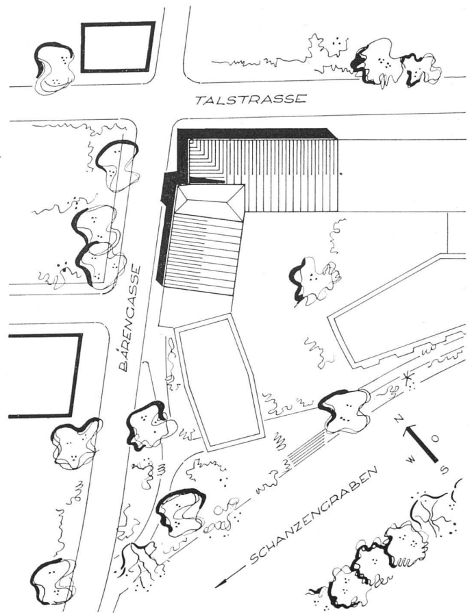
Situation 1:1000 mit projektiertem Hochhaus zwischen Bärengasse und Schanzengraben | Situation, avec l'immeuble tour projeté entre la Bärengasse et le Schanzengraben | Site plan with projected tower house between Bärengasse and Schanzengraben
