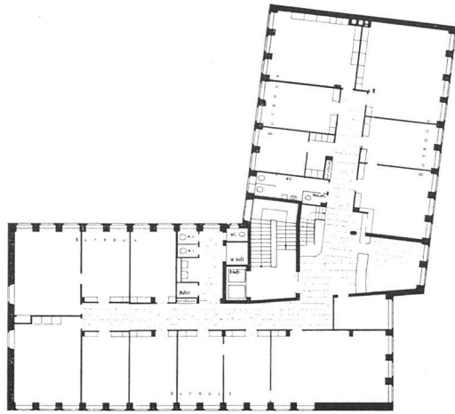
Obergeschosse 1:500 | Etages supérieurs | Upper floors
