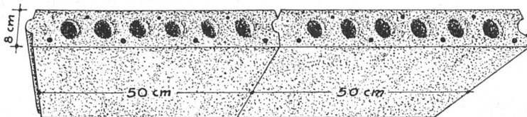
Stegdielendach Wirtschaftliche Pfettenabstände 1.80—2.40 m Maximaler Pfettenabstand 2.65 m
