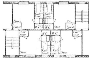
Einzimmerapartment 1:400
