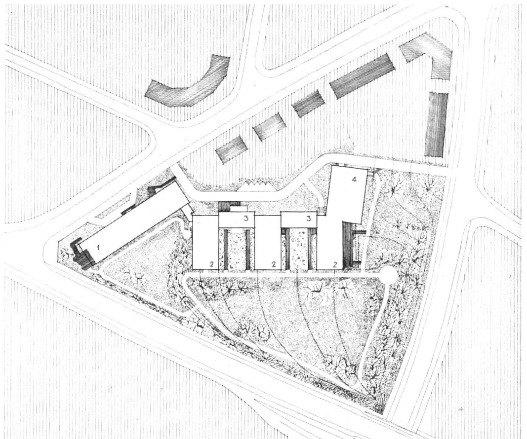
Situation I: 2000 / Plan de situation / Site plan
