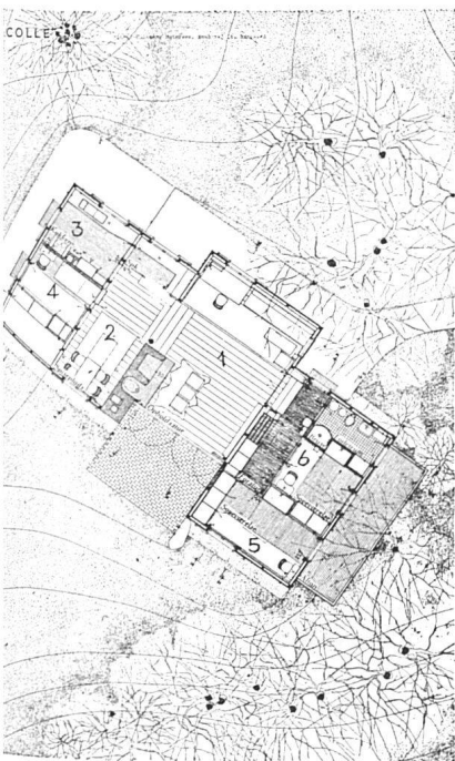
Grundriß 1:350 / Rez-de-chaussée / Ground-floor
