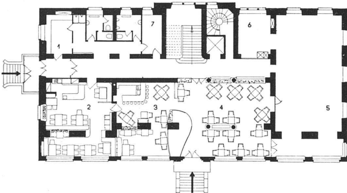
Erdgeschoß vor und nach dem Umbau 1:300 / Le rez-de-chaussée avant et après la transformation / Groundfloor before and after remodelling
