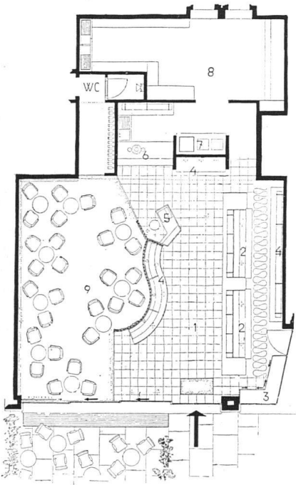
Grundriß 1:200 | Plan
