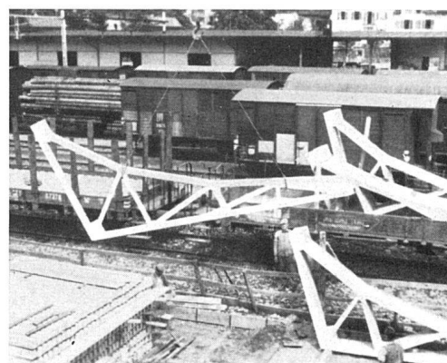
Transport der Binderhälften | Transport des éléments | Transport of the units
