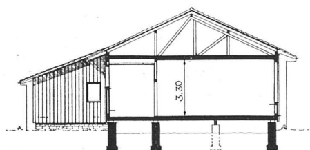
Standard-Pavillon (Ahornstraße, In der Probstei) Grundriß und Schnitt 1:300 / Pavillon standard, plan et coupe / Standard classroom wing; plan and section
