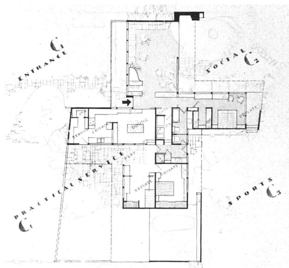
Grundriß 1:400 | Plan 1:400
