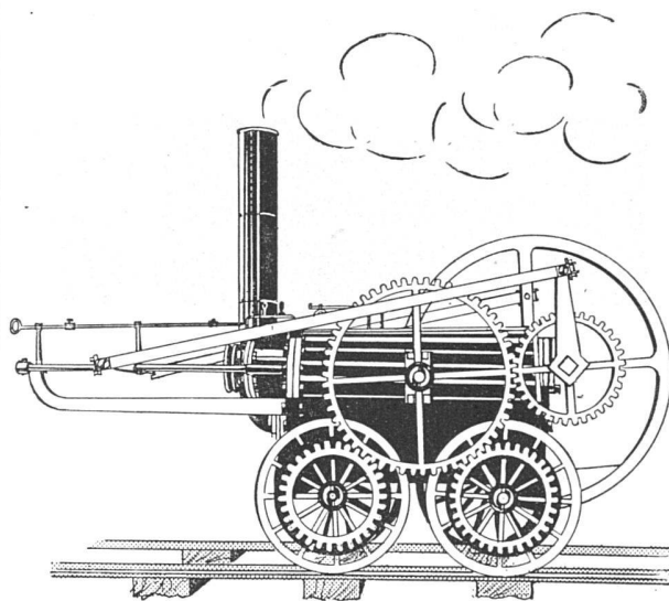
Älteste Schienenlokomotive von Trevithick, 1803
