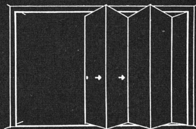
Harmonika-Falttüre Detail 1:1, Nr. 21
