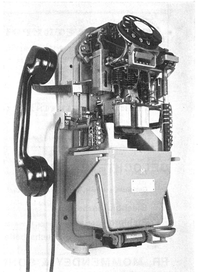
(Kassierstation Typ M geöffnet)
