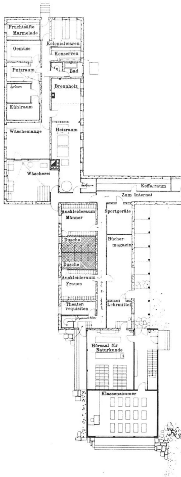
Grundriss 1 : 500 Untergeschoss und Erdgeschoss
