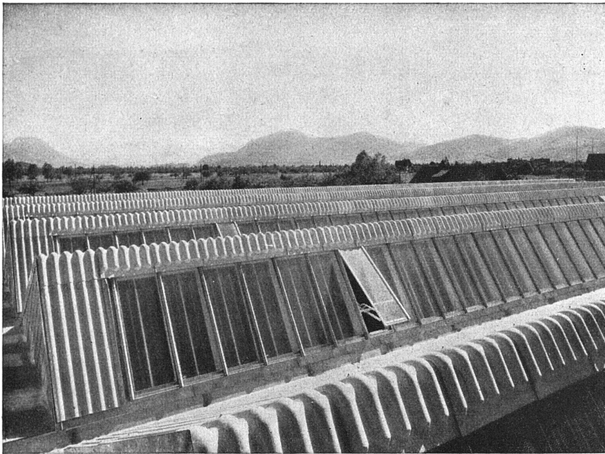
Sheddächer des Fabrikneubaus der Verkaufs-A. G. Heinrich Wild, Geodätischer Instrumente, Heerbrugg
