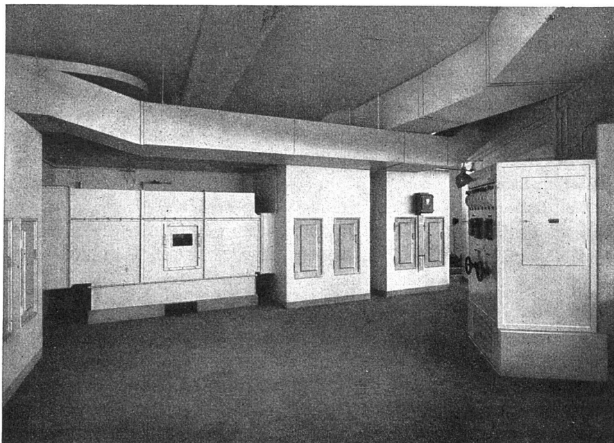
Luftkonditionierungsanlage für den neuen Rotationsmaschinensaal der Buchdruckerei Berichthaus, Zürich, verbunden mit kompletter Lüftung der Garage, Wagenwäscherei und des Speditionsraumes
