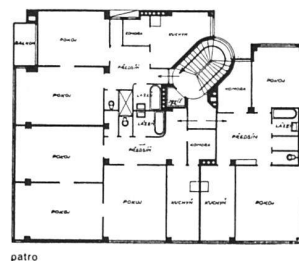
Geschäfts- und Miethaus in Prag-Bubeneč Architekten Arnošt Muhlstein und Victor Fürth
