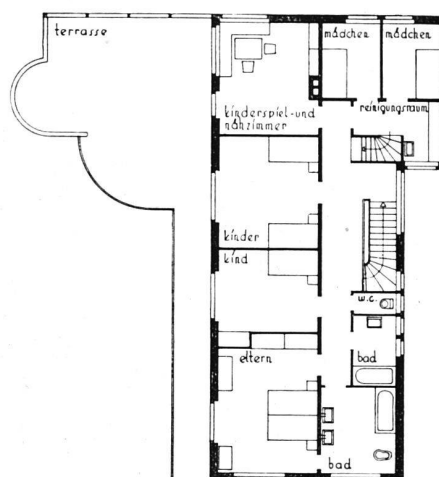
Obergeschoss 1 : 300
