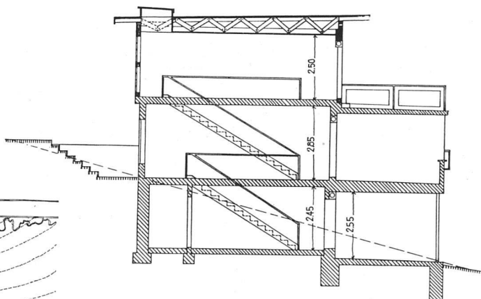
oben: Querschnitt 1:200
