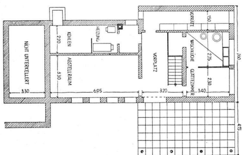
Keller, Erdgeschoss, Obergeschoss, Grundrisse 1:300
