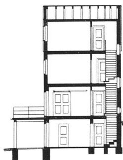
Schnitt 1:300
