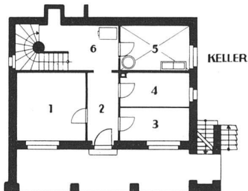
Schnitt und Grundrisse 1:300
