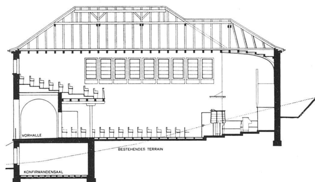
Längsschnitt 1:300
