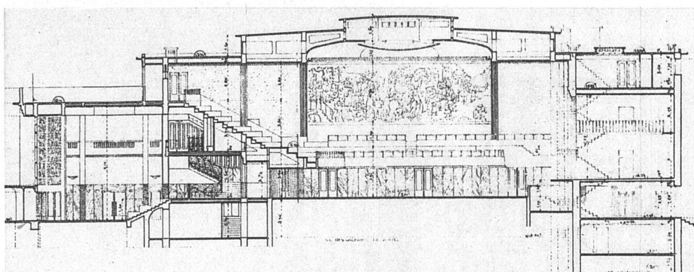
Coupe longitudinale 1:400
