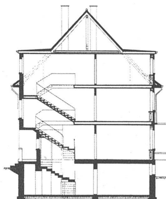
Schnitt
