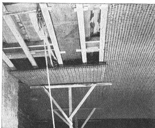
Rissfreie Drahtziegeldecken
