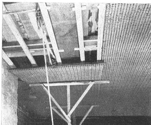
Rissfreie Drahtziegeldecken
