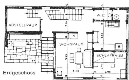
Grundrisse 1:200
