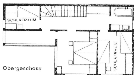
Grundrisse 1:200
