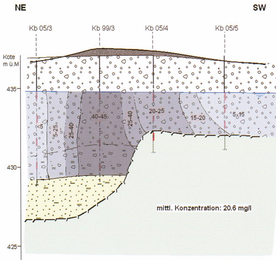
Fig. 20: Räumliche Verteilung der CKW-Konzentrationen in der Kontrollebene (Stand 20.2.2013). Die Zahlen in der Figur geben die pro ausgeschneider Flächeneinheit mittlere CKW-Konzentration in µg/l wider.
