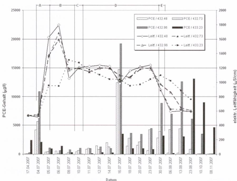
Fig. 9: Verlauf des PCE-Gehalts und der elektrischen Leitfähigkeit während der Injektion (Pilotphase) ca. 6 m abstromseitig der Injektionsstelle Kb 04/2. Multilevel-Probeentnahmekompartimente 25, 50, 75 und 100 cm ab Stauer (432.48, 432.73, 432.96 und 433.23 m ü. M.). Phase A: Injektion/Extraktion alternierend; Phase B: nur Extraktion; Phase C: kontinuierliche Injektion; Phase D: nur Extraktion [Zirkulation ohne Injektion].
