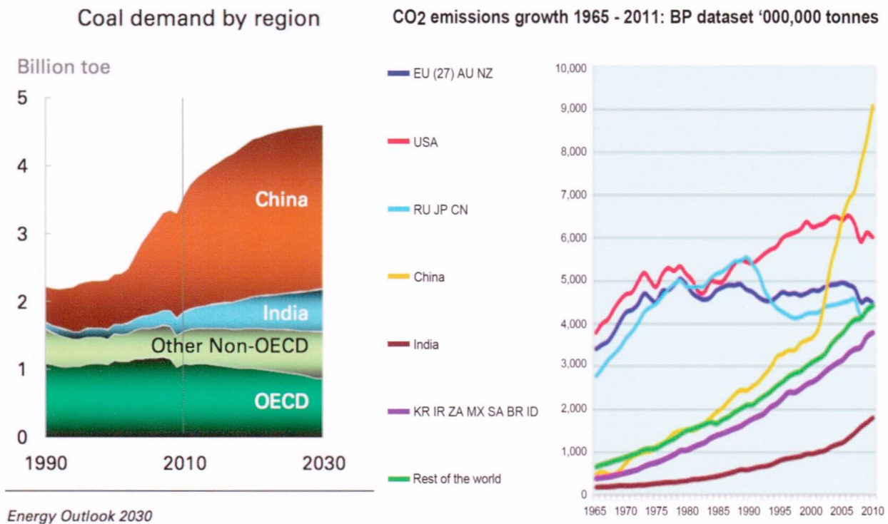
Fig. 6: Der am schnellsten wachsende fossile Energieträger: Kohle und die Auswirkung auf den CO 2 -Ausstoss. Der rapide Anstieg der CO 2 -Emissionen in China und in anderen Schwellenländern ist vor allem die Folge des stark steigenden Kohlenverbrauchs. Noch bedenklicher als CO 2 ist aber die Luft-Schadstoffbelastung in den Städten. Nur eine Substitution durch Gas kann diese Probleme in den kommenden Jahrzehnten mildern (Quelle IEA, World Energy Outlook 2013).
