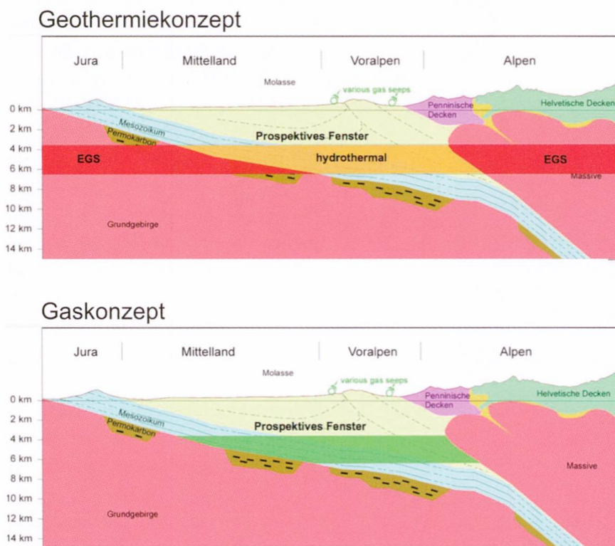
Fig. 2: Synergie zwischen Geothermie und Kohlenwasserstoff-Exploration. Die Tiefenbereiche sind dieselben. Die hydrothermale Geothermie exploriert teilweise dieselben stratigraphischen Horizonte, nur die Enhanced Geothermal Systems (EGS) erforschen mit dem Kristallin neue stratigraphische und lithologische Ziele.
