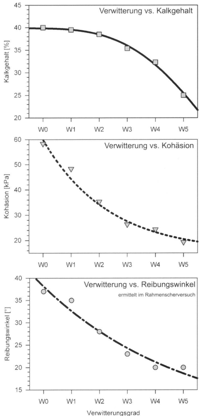
Fig. 8: Abnahme der Bodenkennwerte mit zunehmender Verwitterung.
