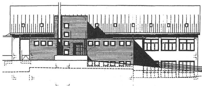
Plan Werkstattneubau im Gehörlosendorf in Turbenthal
