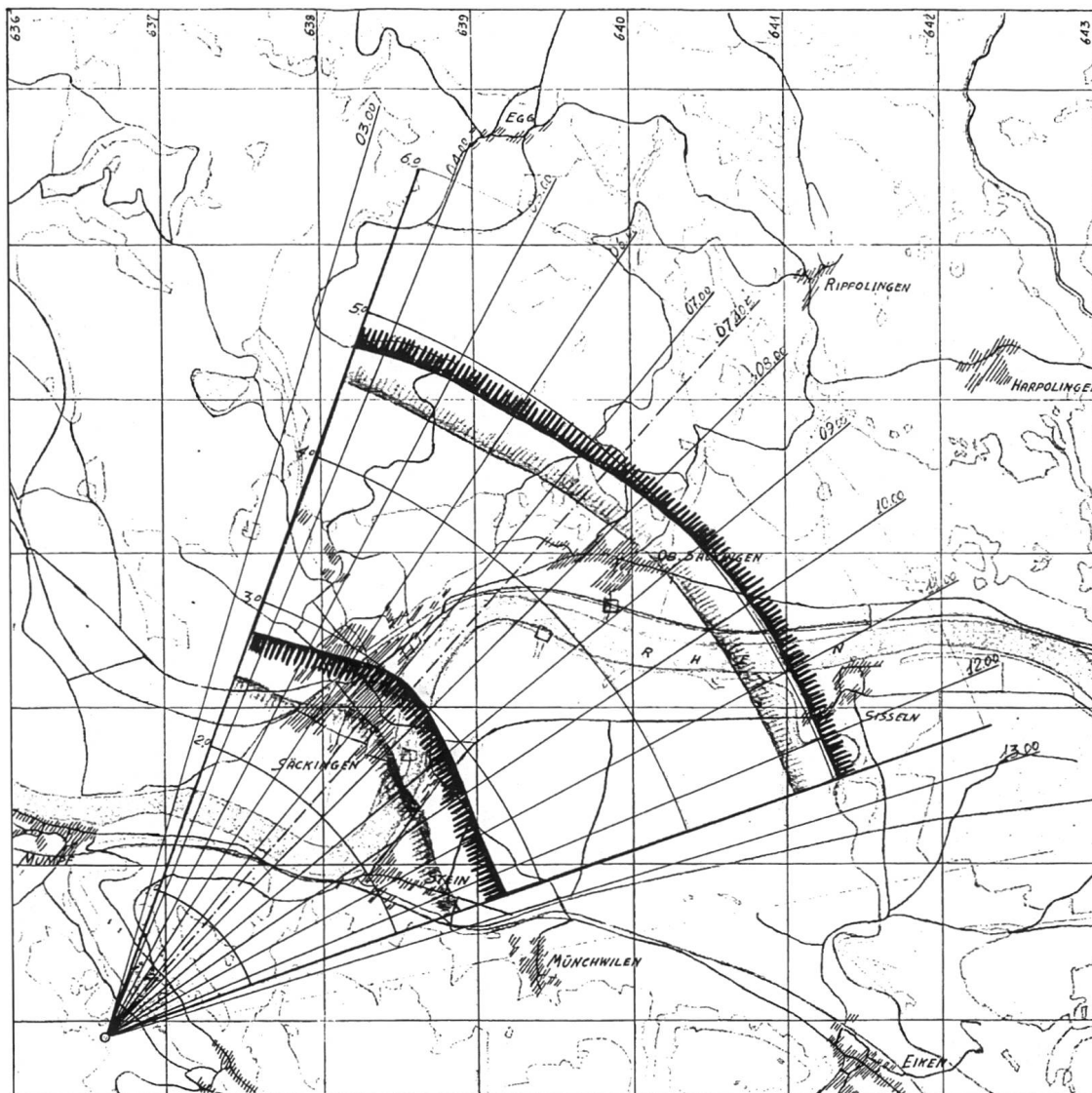
Abb. 12: Artilleriewerk «Obermumpf»: Wirkungsmöglichkeit mit 7,5-cm-Gebirgs- kanone (Kurz- und Langschuss mit Stahlgranaten- Doppelzünder und -Momentanzünder, 1941. (BAB)
