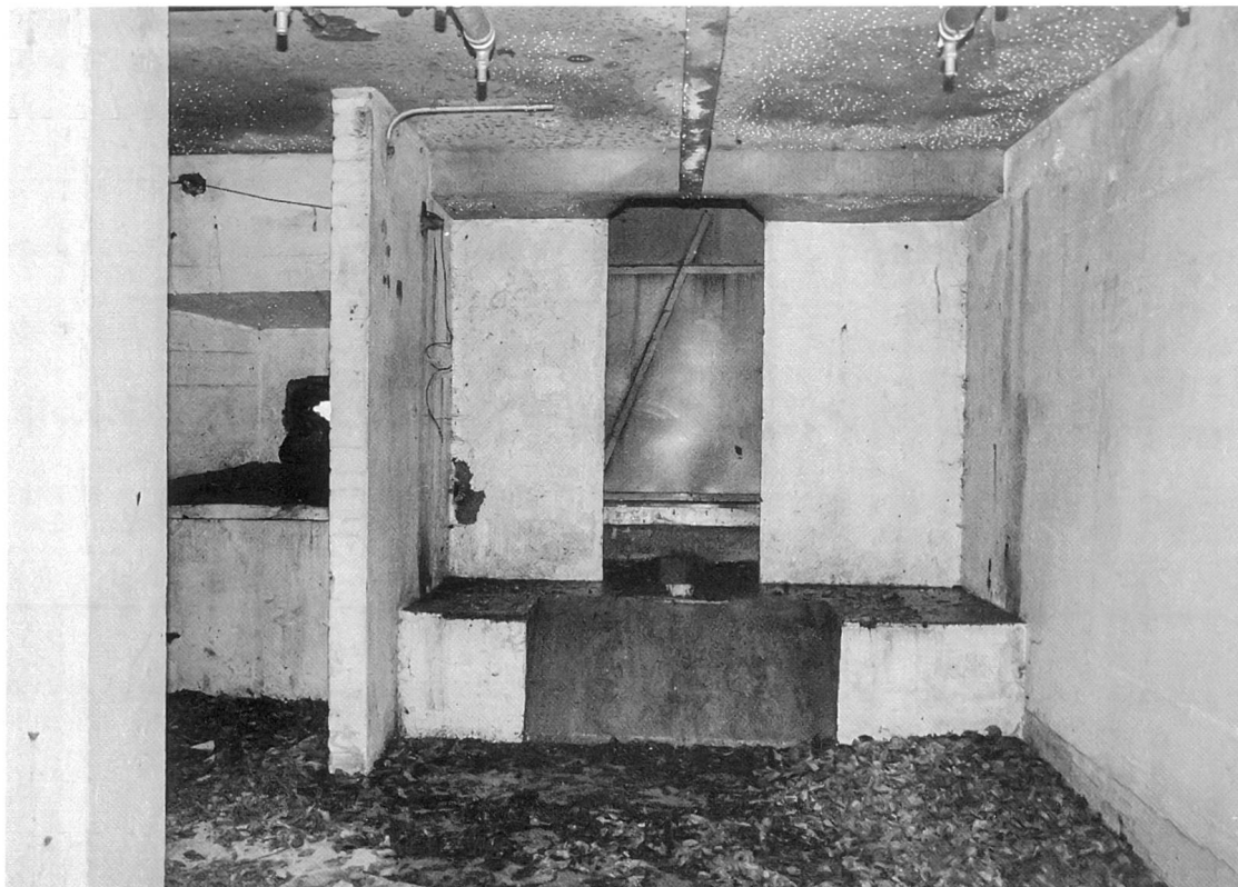
Abb. 6: Artilleriewerk «Zeihher Homberg»: Geschützkaferne 2 mit geschlossener Scharfe. Links Scharfe für Beobachter, evtl. für Infanteriewaffen, 1999. (Foto Jörn Maurer)
