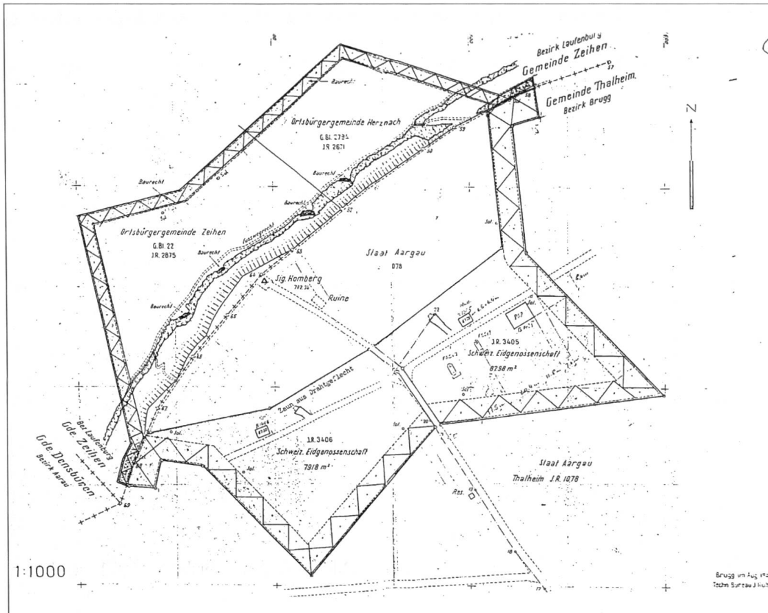
Abb. 7: Die Aussenanlagen des Artilleriewerkes «Zeiher Homberg»: Stacheldrahtumzäu- nung, Baracken usw., die alle beseitigt sind. (Akten FWK)
